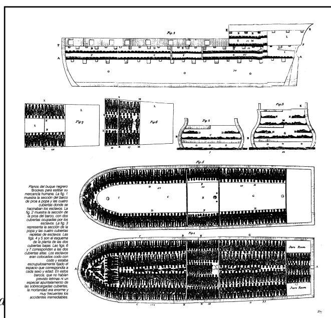
Plànols del vaixell negrer Brookeon es mostra com col·loquen els esclaus.
